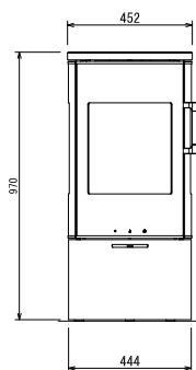
正面図
