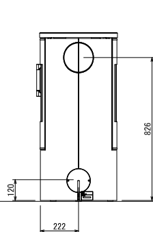
背面図
