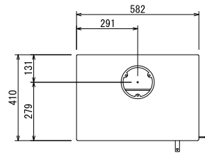
平面図
