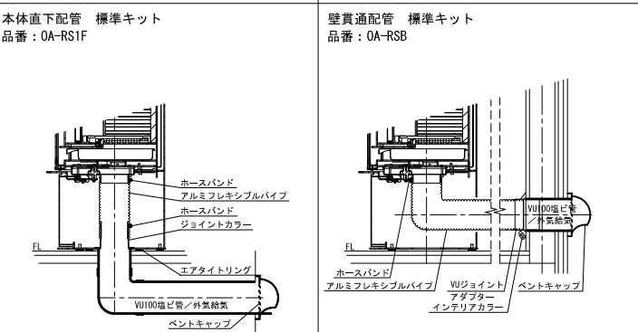
外気導入キット取付図
