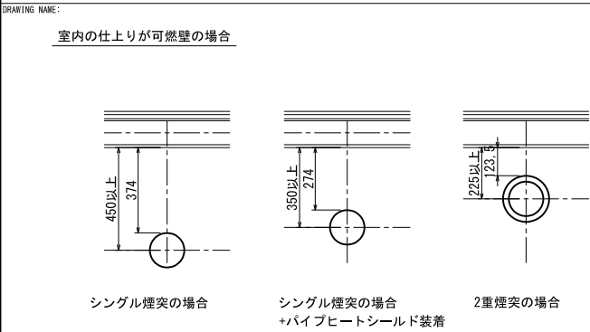
煙突の推奨離隔距離
